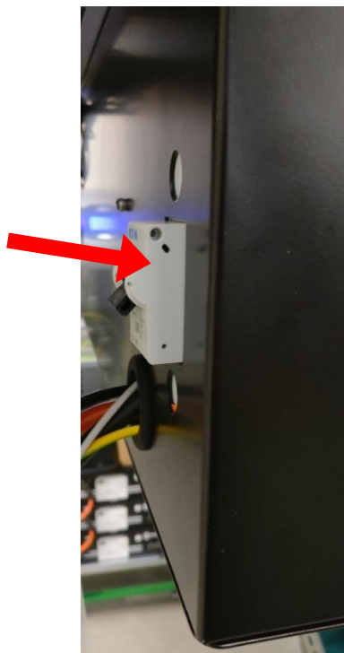
Figura 84 – Abbassare la leva dell'interruttore QB1 per attivare il M.Store
