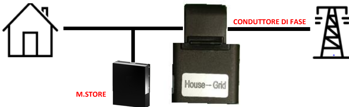
Figura 41 - CT: rispettare il verso di installazione
