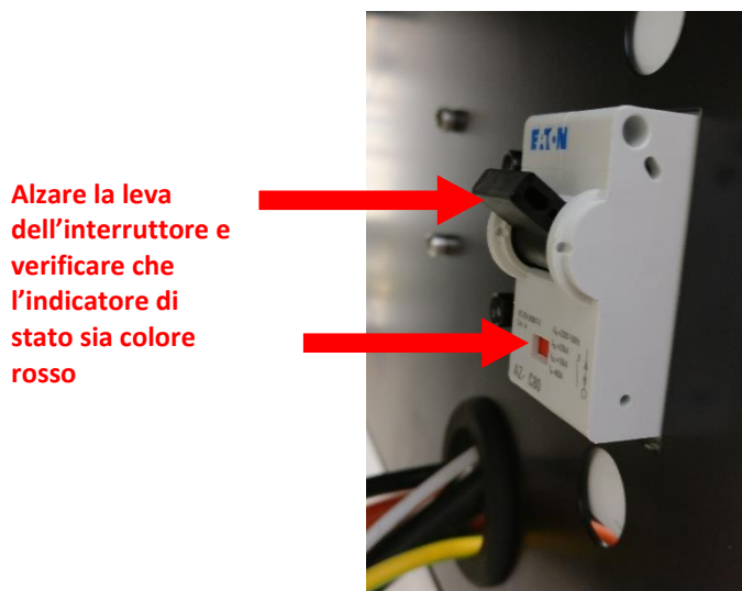
Figura 58 – Sollevare la leva dell'interruttore QB1
