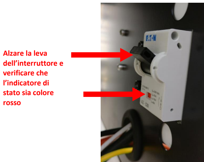
Figura 85 – Sollevare la leva dell'interruttore QB1 per attivare il M.Store
