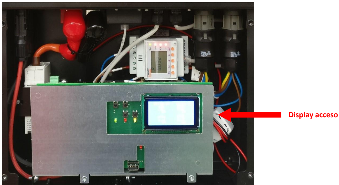
Figura 60 – Display acceso
