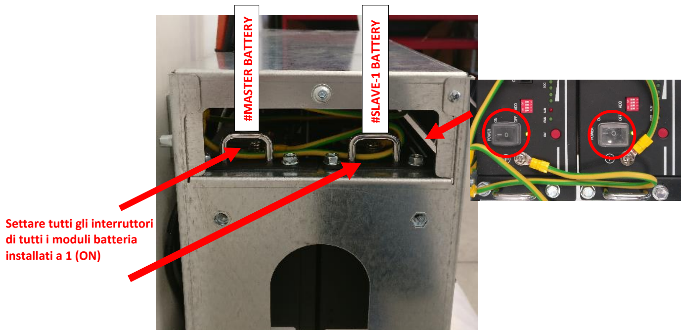
Figura 56 – Posizionare su “1” tutti gli interruttori di tutti i moduli batteria installati sul sistema di accumulo
