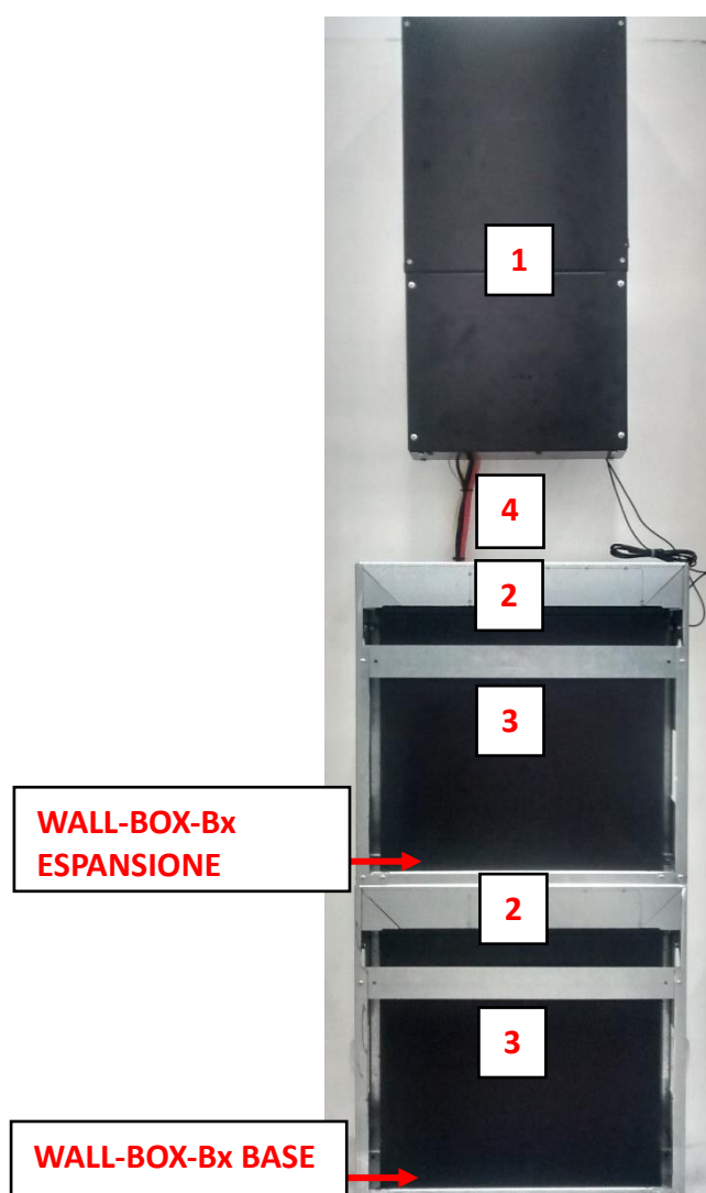
Figura 1 – Composizione sistema M.Store
