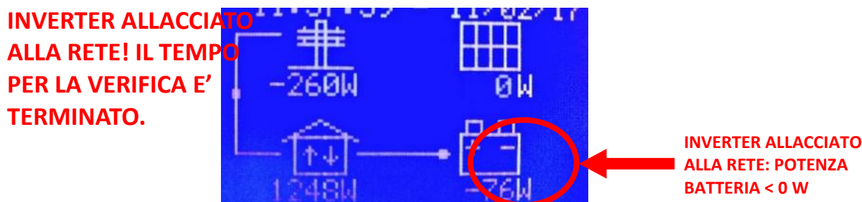
Figura 64 - Inverter allacciato alla rete
