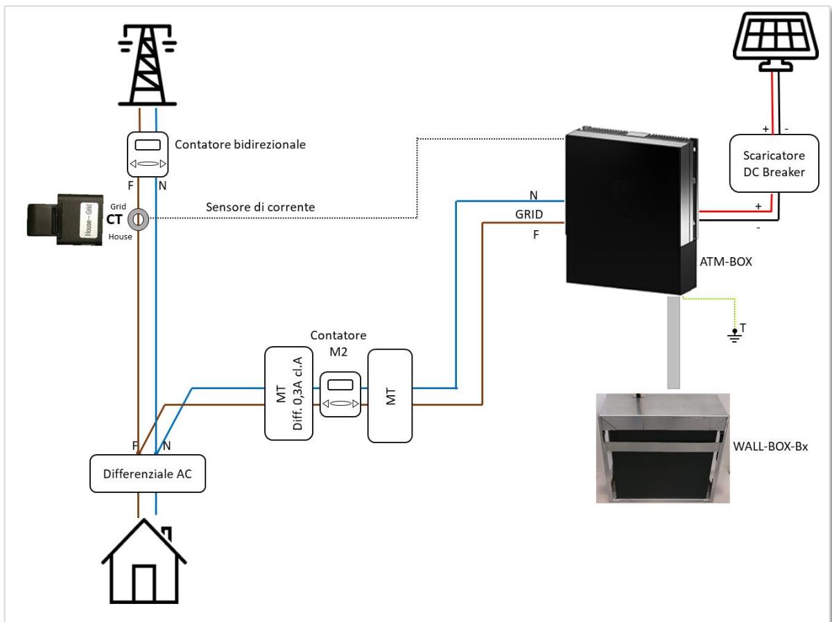
Figura 45 - Sensore CT: rispettare il verso di installazione
